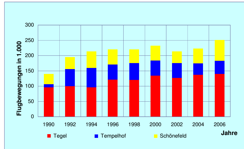
Abb. 3-18: Entwicklung der Flugbewegungen insgesamt
